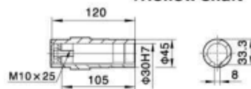
FA37/FAF37/FAZ37空心轴 /Hollow shaft
